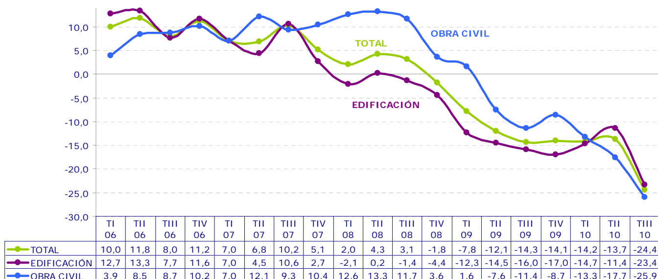
Gráfico 1. Crecimiento trimestral interanual del Índice Coyuntural de la Construcción corregido de la C.A. de Euskadi. Total, Edificación y Obra Civil. (%)
